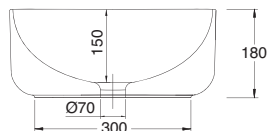
SEZIONE A-A
